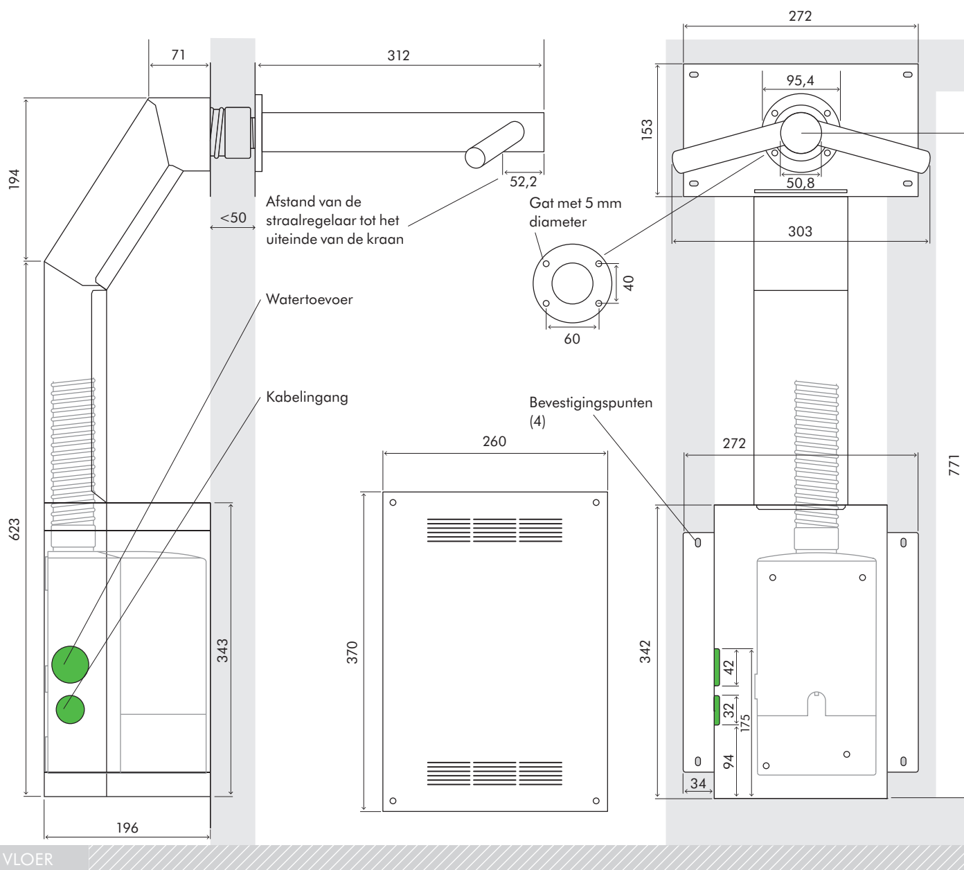
ZIJAANZICHT
